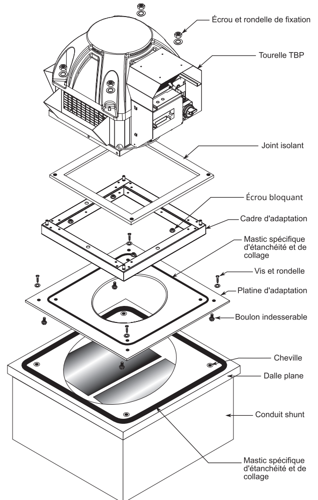
Vue éclatée d'une tourelle TBP sur dalle plane conservée avec cadre et platine d'adaptation
