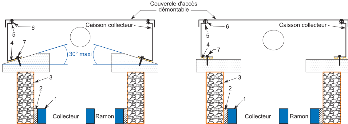
Coupe verticale d'un caisson collecteur en applique sur dalle plane conservée
