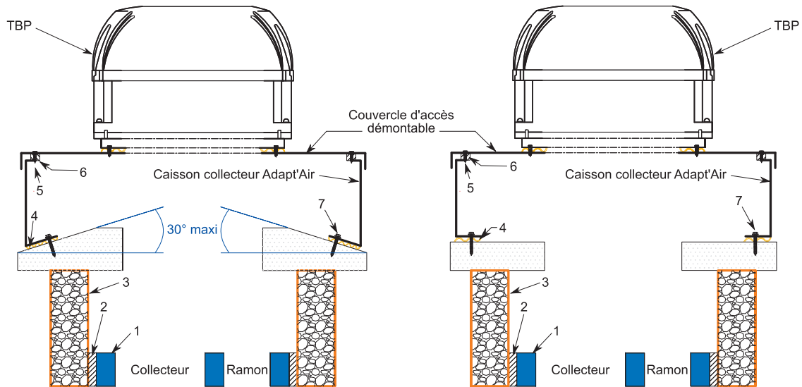
Coupe verticale d'un caisson collecteur Adapt'Air en applique sur dalle plane conservée
