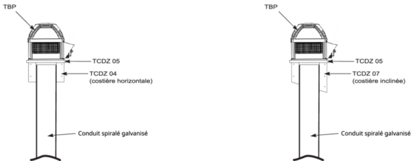
Figure 23 – Mise en œuvre d'une tourelle d'extraction sur conduit circulaire neuf
