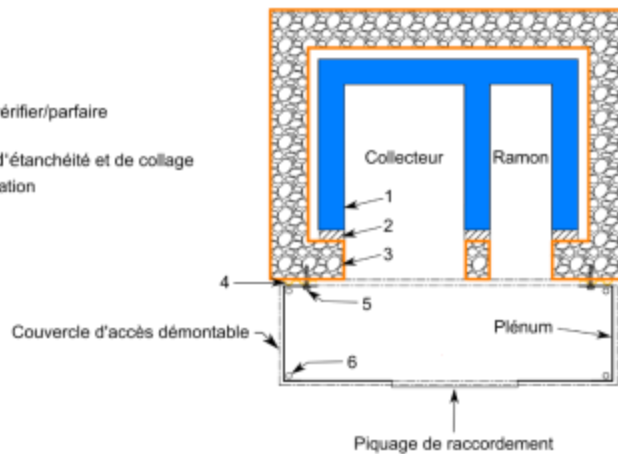
Figure 21 - Coupe horizontale d'un plénum sur souche
