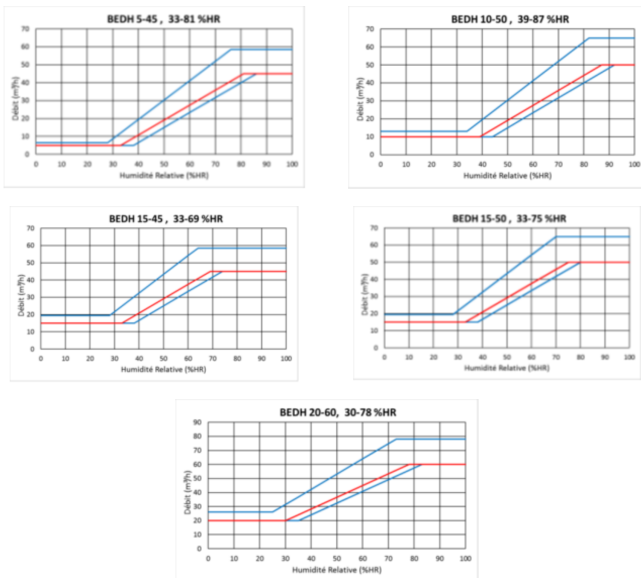
Figure 4 – Courbes hygroaérauliques des bouches d'extraction hygroréglables
