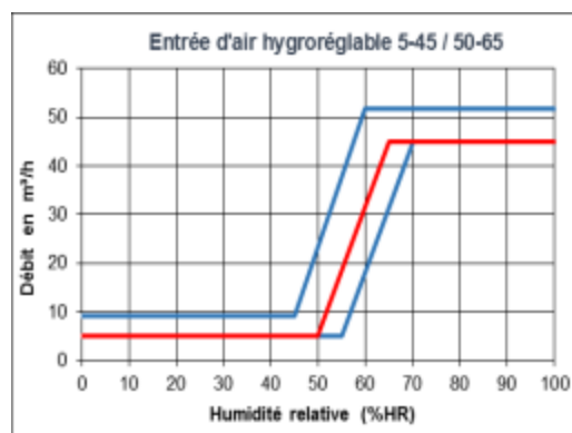
Figure 1 – Entrée d'air hygro-réglable 5-45 / 50-65 (HY) Caractéristiques hygroaéroulques pour une différence de pression de 20 Pa
