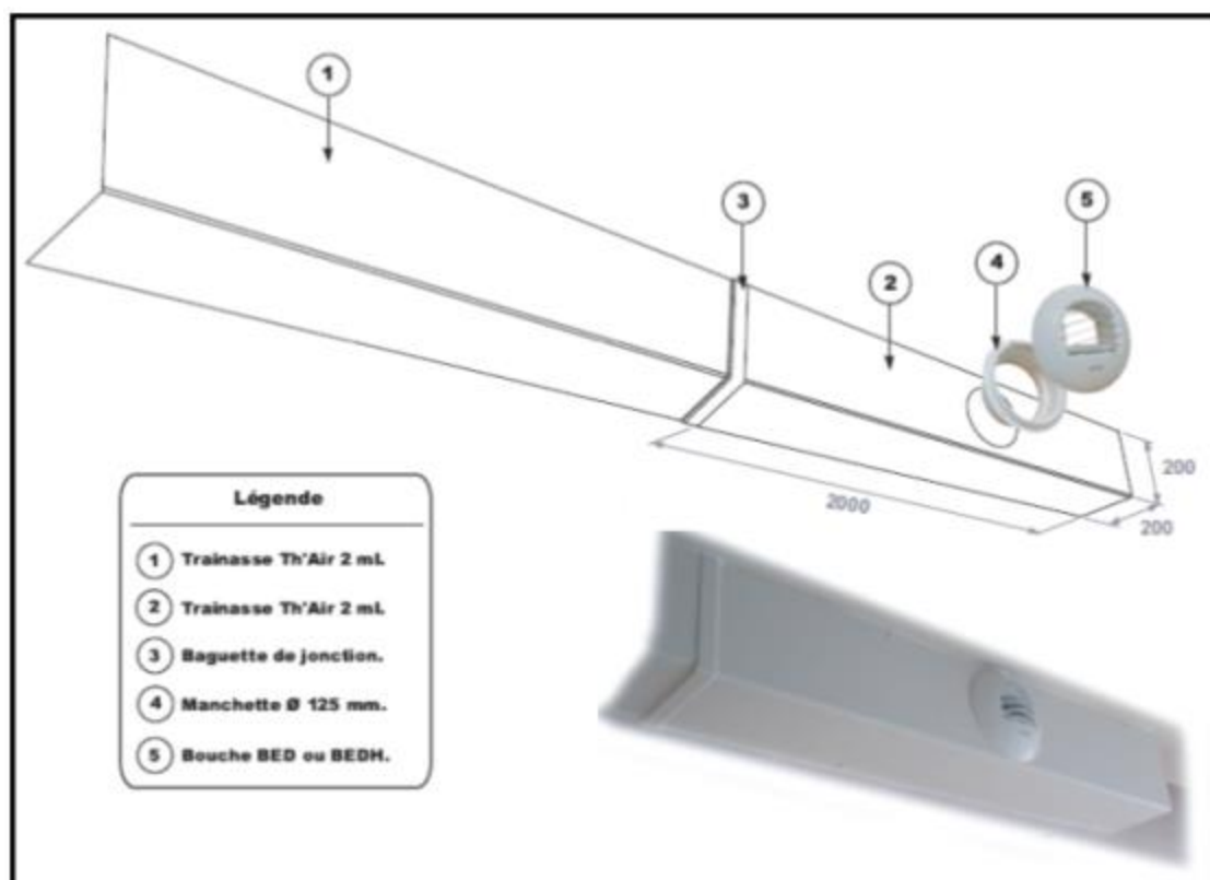
Figure 9 – Caractéristiques dimensionnelles de la trainasse horizontale Th'Air
