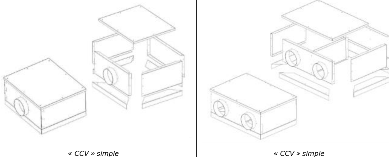
Figure 12 – Caisson collecteur « CCV »
