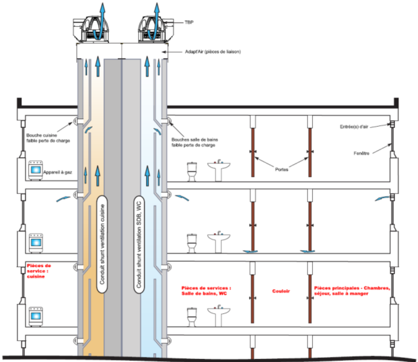
Figure 27 – Systèmes Novat'Air® Hygro : schéma de principe avec réseau horizontal en toiture-terrasse
