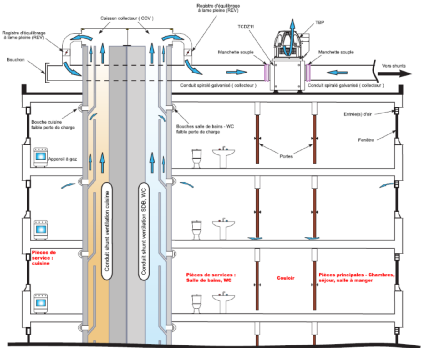
Figure 26 – Systèmes Novat'Air® Hygro : schéma de principe sans réseau horizontal
