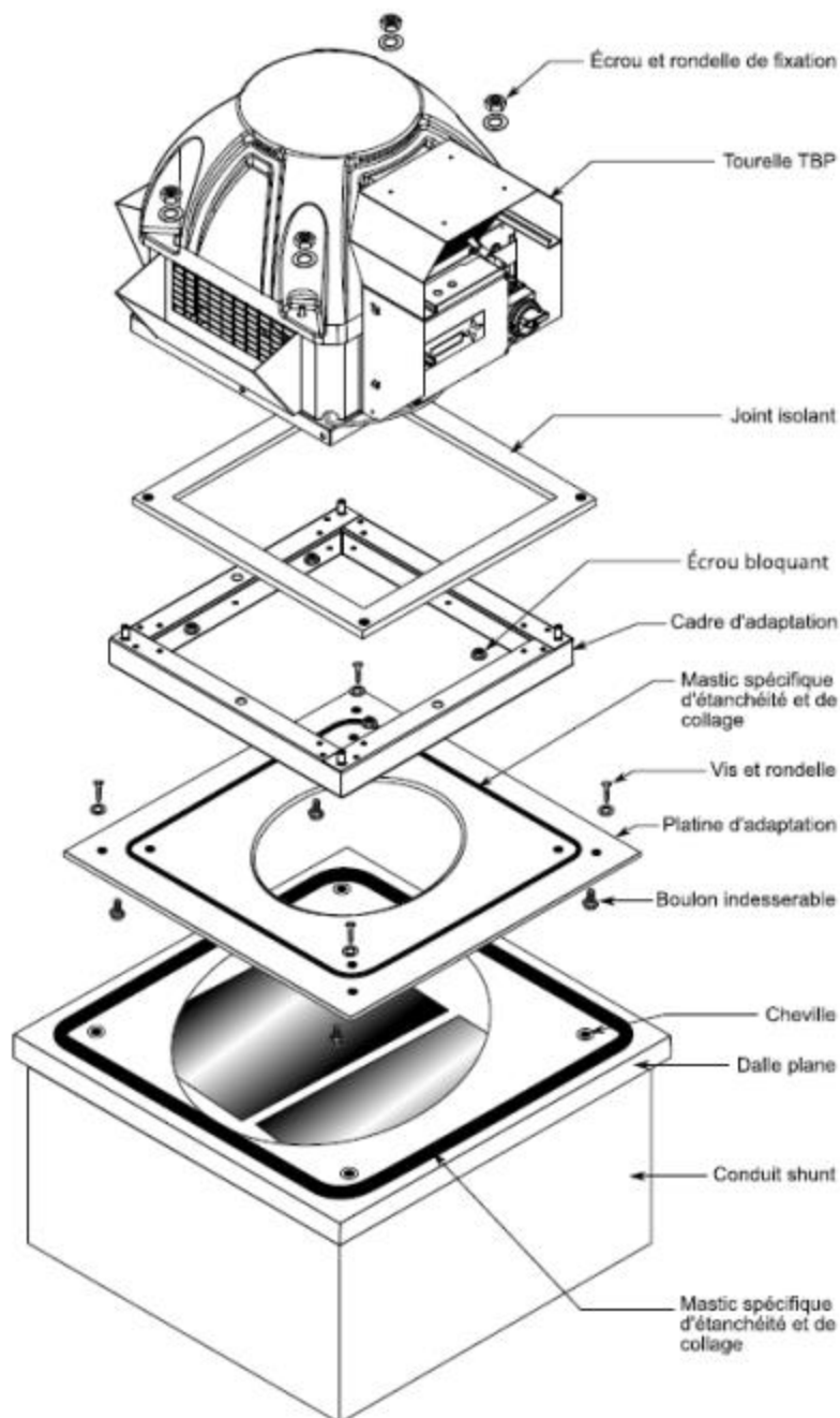
Figure 25b – Mise en œuvre d'une tourelle sans « Adapt'Air » - Avec platine d'adaptation
