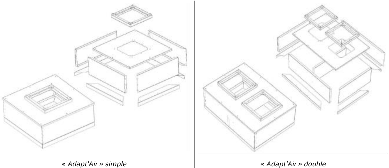
Figure 13 - Caisson collecteur « Adapt'Air »
