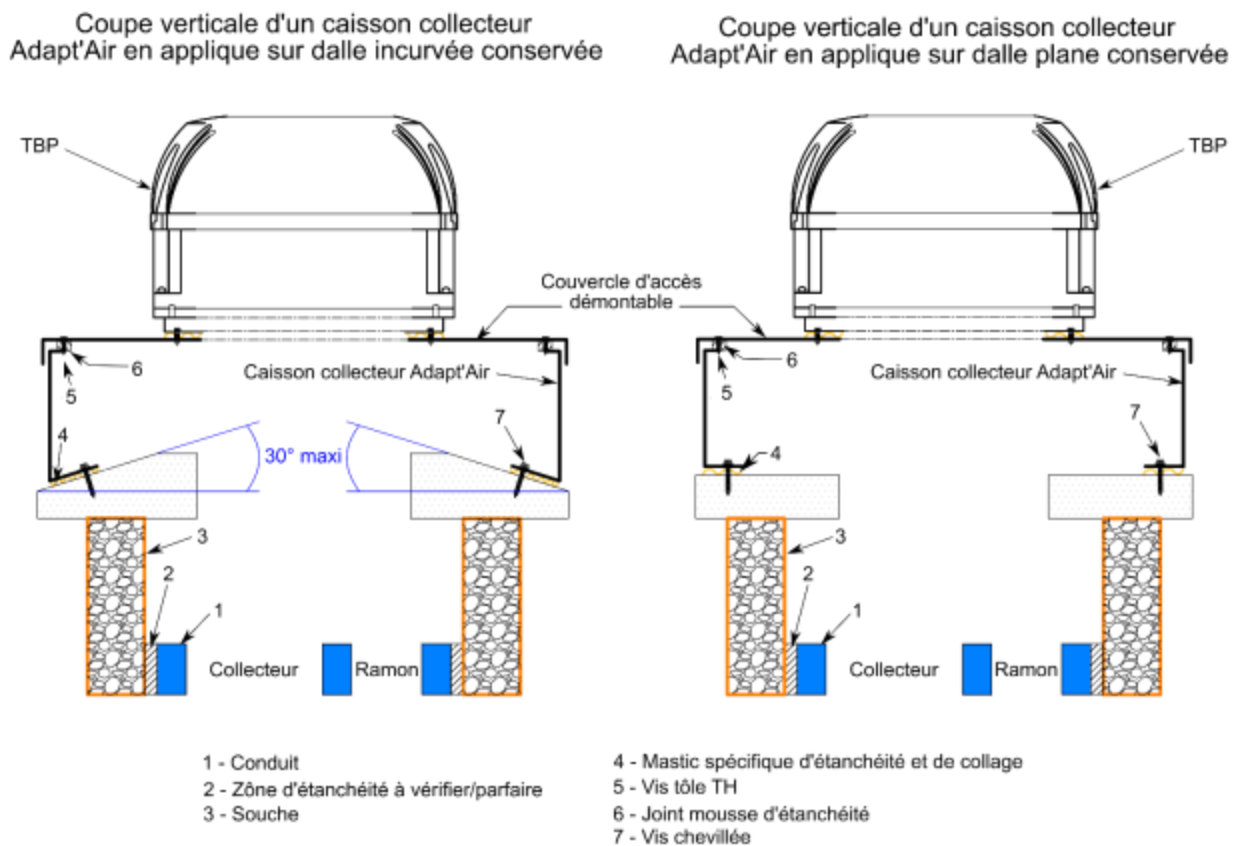
Figure 20 - Coupe verticale d'un caisson collecteur Adapt'Air en applique (sans goutte d'eau) sur dalle existante
