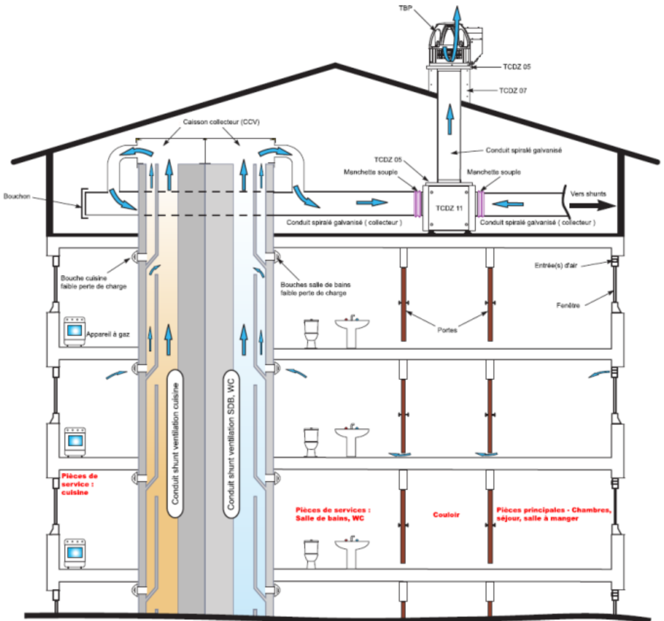
Figure 28 – Systèmes Novat'Air® Hygro : schéma de principe avec réseau horizontal en combles accessibles
