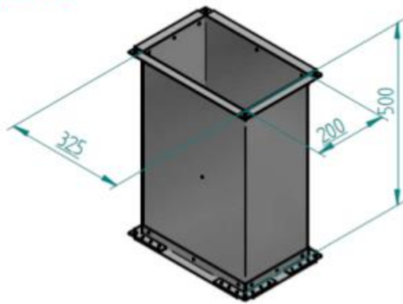
Elément liaison Type CSM Elément n°2
