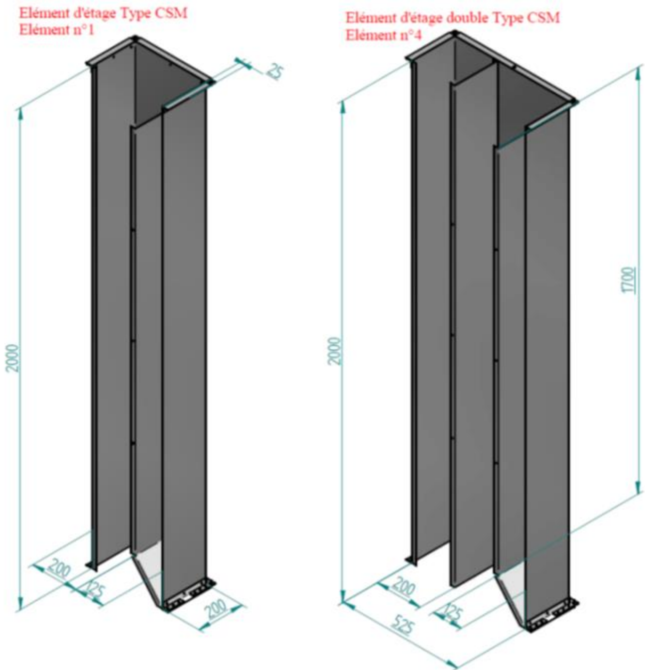
Caractéristiques dimensionnelles des éléments d'étages type CSM
