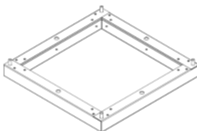
Figure 7 – Cadre métallique intégré aux tourelles d'extraction
