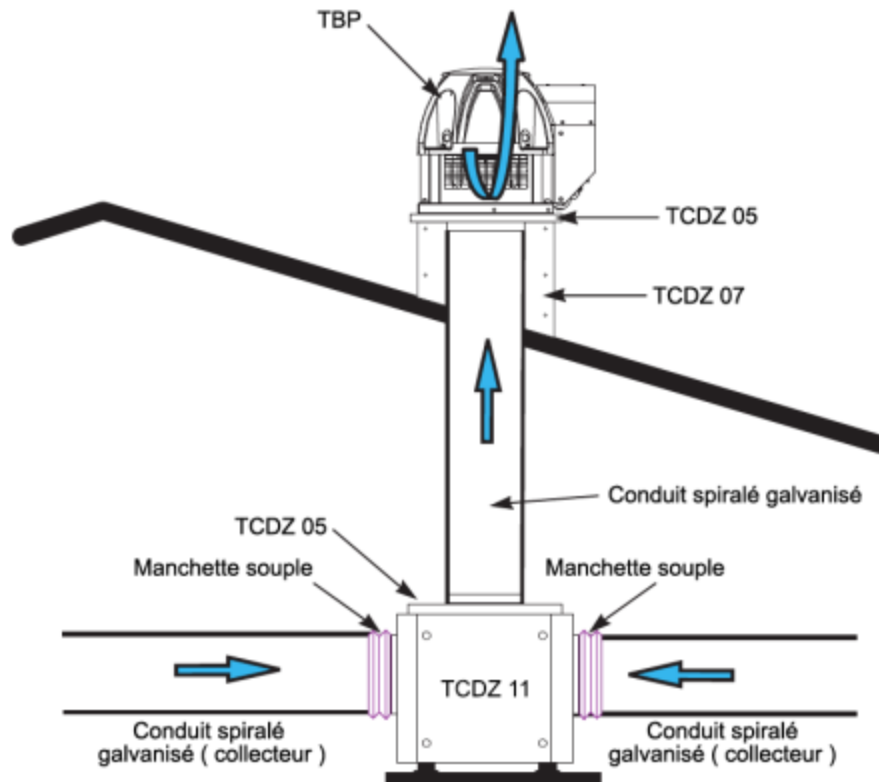
Figure 24 – Mise en œuvre d'une tourelle d'extraction sur toiture inclinée
