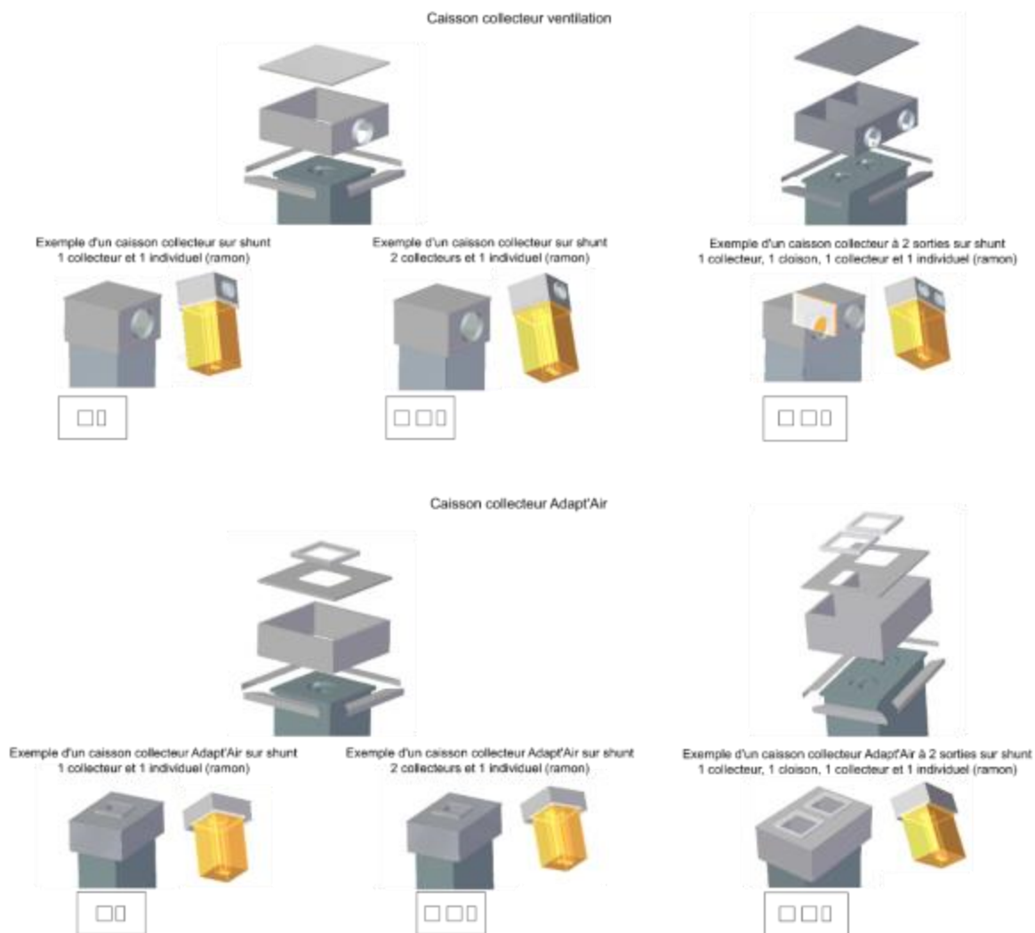
Figure 15 – Schémas de principe en cas de conservation de la dalle existante
