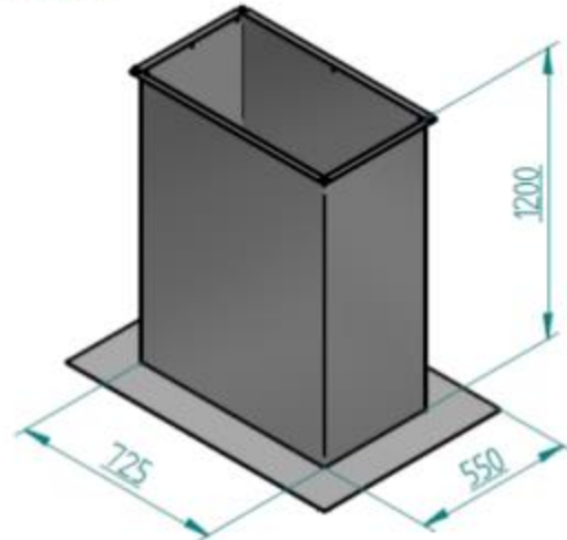
Elément sortie de toiture Type CSM Elément n°3
