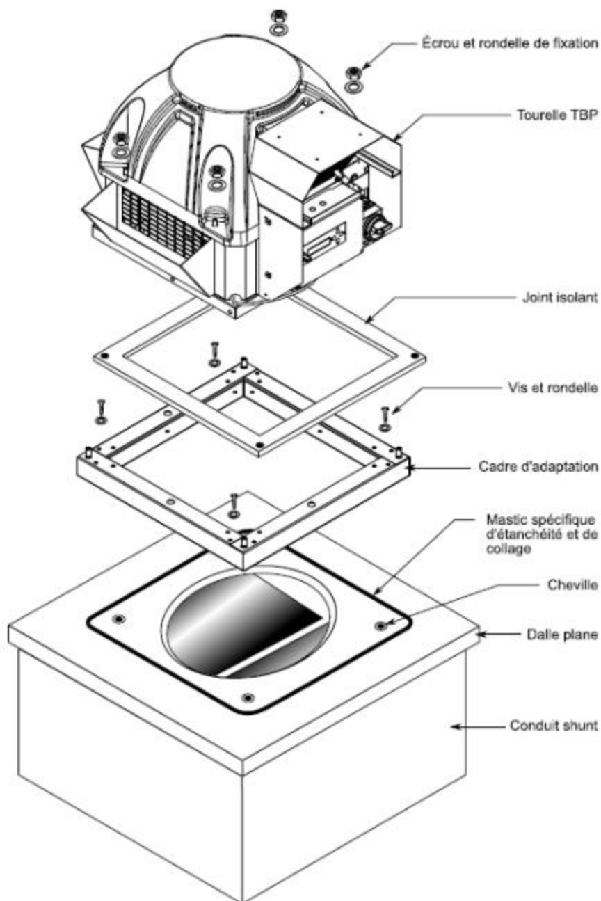
Figure 25a - Mise en œuvre d'une tourelle sans « Adapt'Air » - Sans platine d'adaptation
