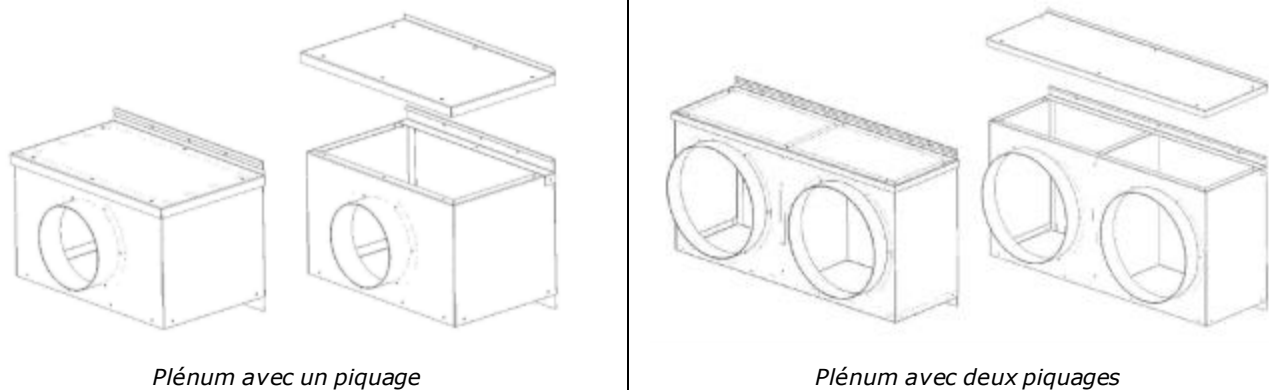
Figure 14 - Visuels de plénums
